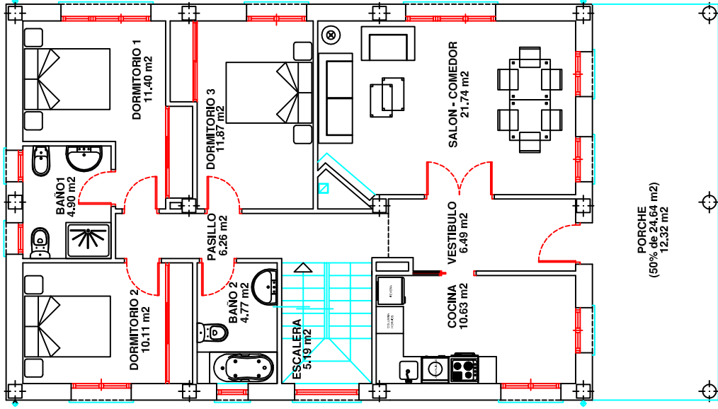
PLANTA BAJA
