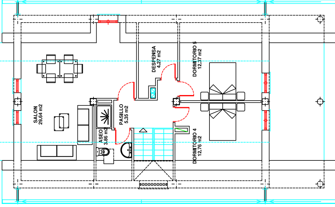
PLANTA BAJOCUBIERTA
